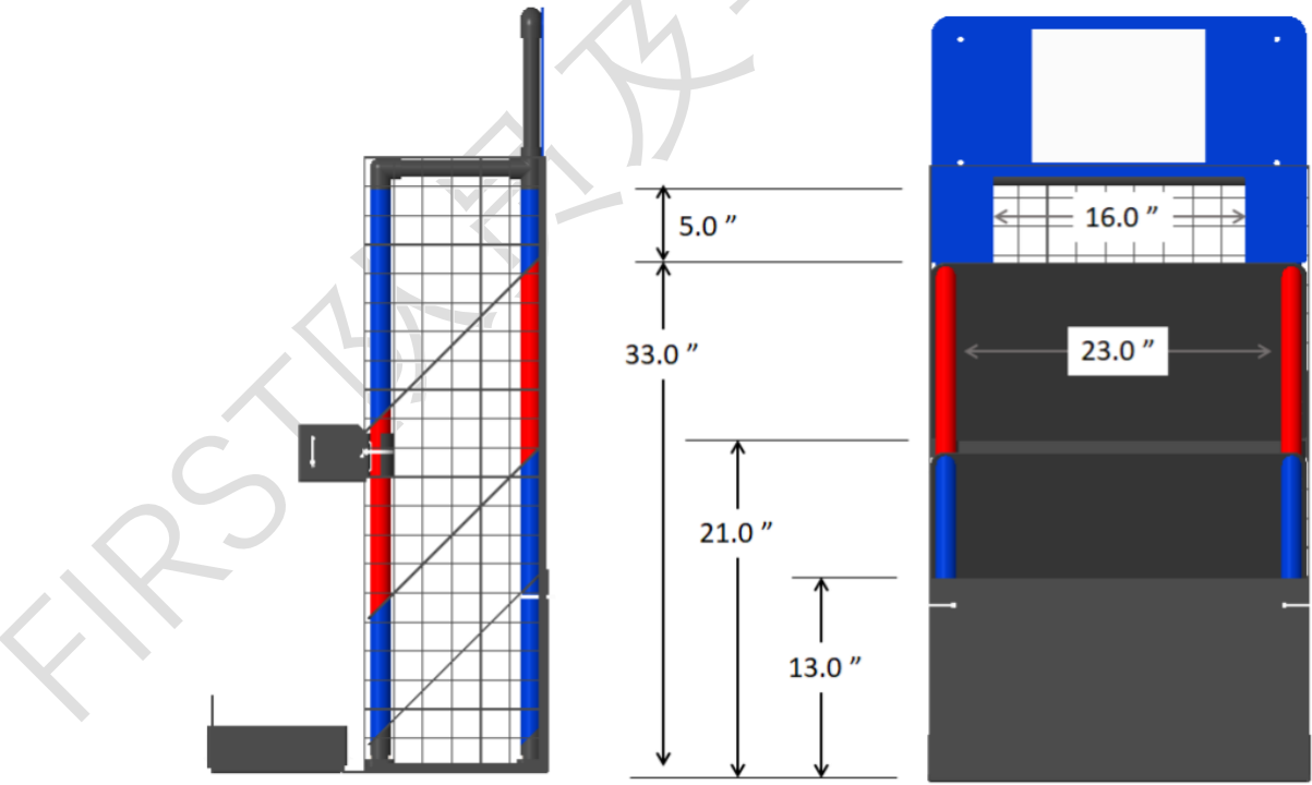
B-2 塔的尺寸
